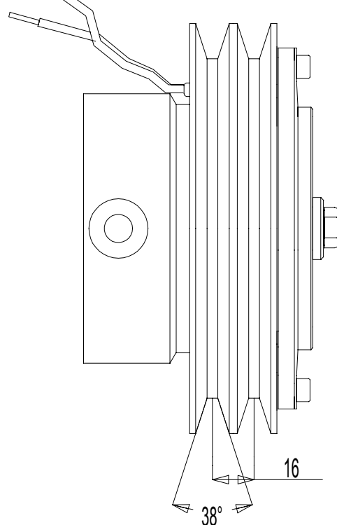
N°2 GOLE SEZ A DIAMETRO PRIMITIVO: Dp=145mm
