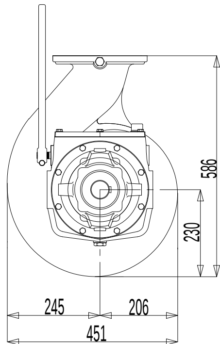
Flangia di mandata
