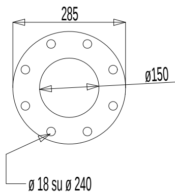
Dimensioni estremità albero
