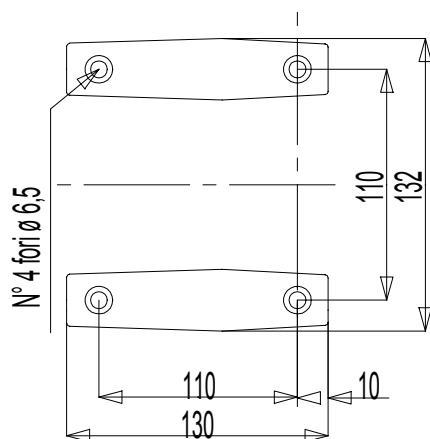
Dimensioni piedi
