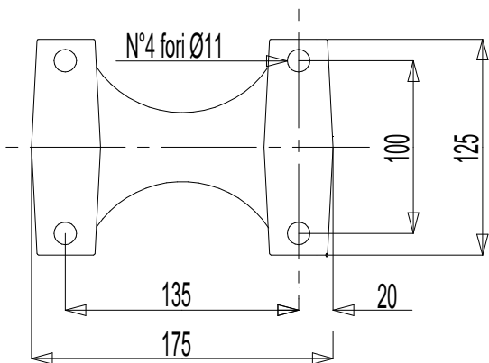
Dimensioni piedi
