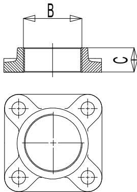
Controflange filettate
