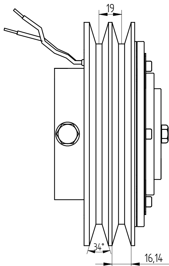
N°2 GOLE SEZ SPB DIAMETRO PRIMITIVO: Dp=180mm
