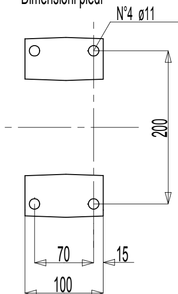
Dimensioni piedi
