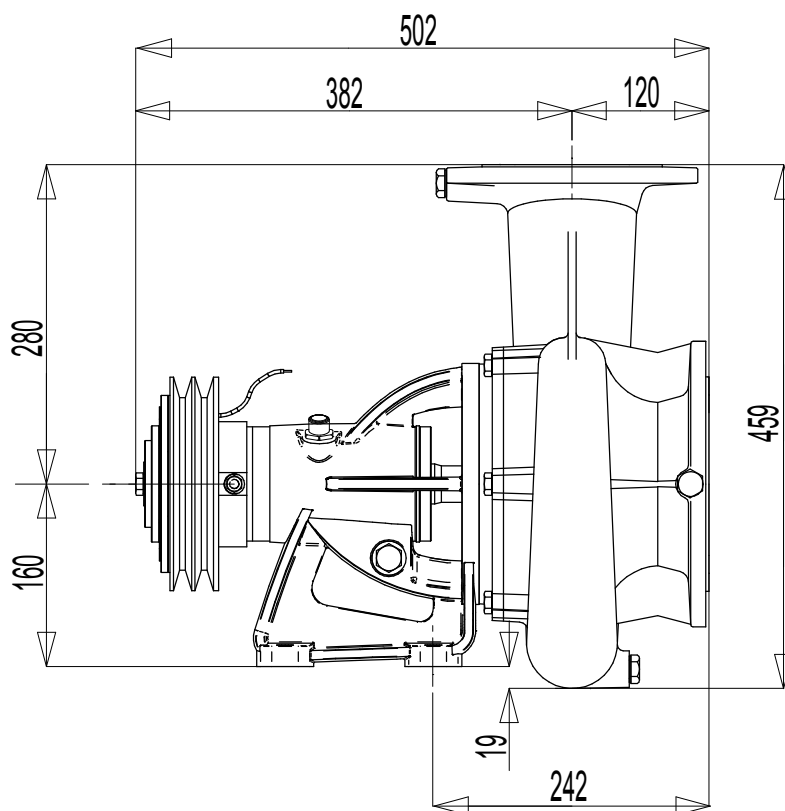
N°2 GOLE SEZ. SPB DIAMETRO PRIMITIVO: Dp=180mm
