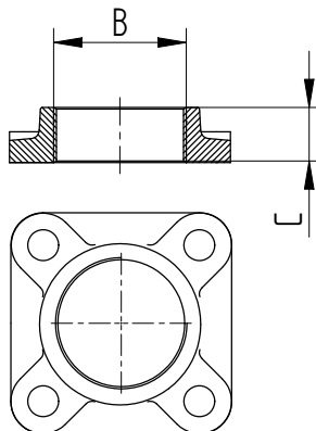
Controflange filettate
